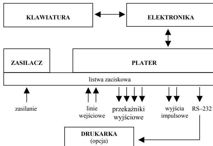
Rysunek 2. Schemat blokowy koncentratora miniSRE-1.
