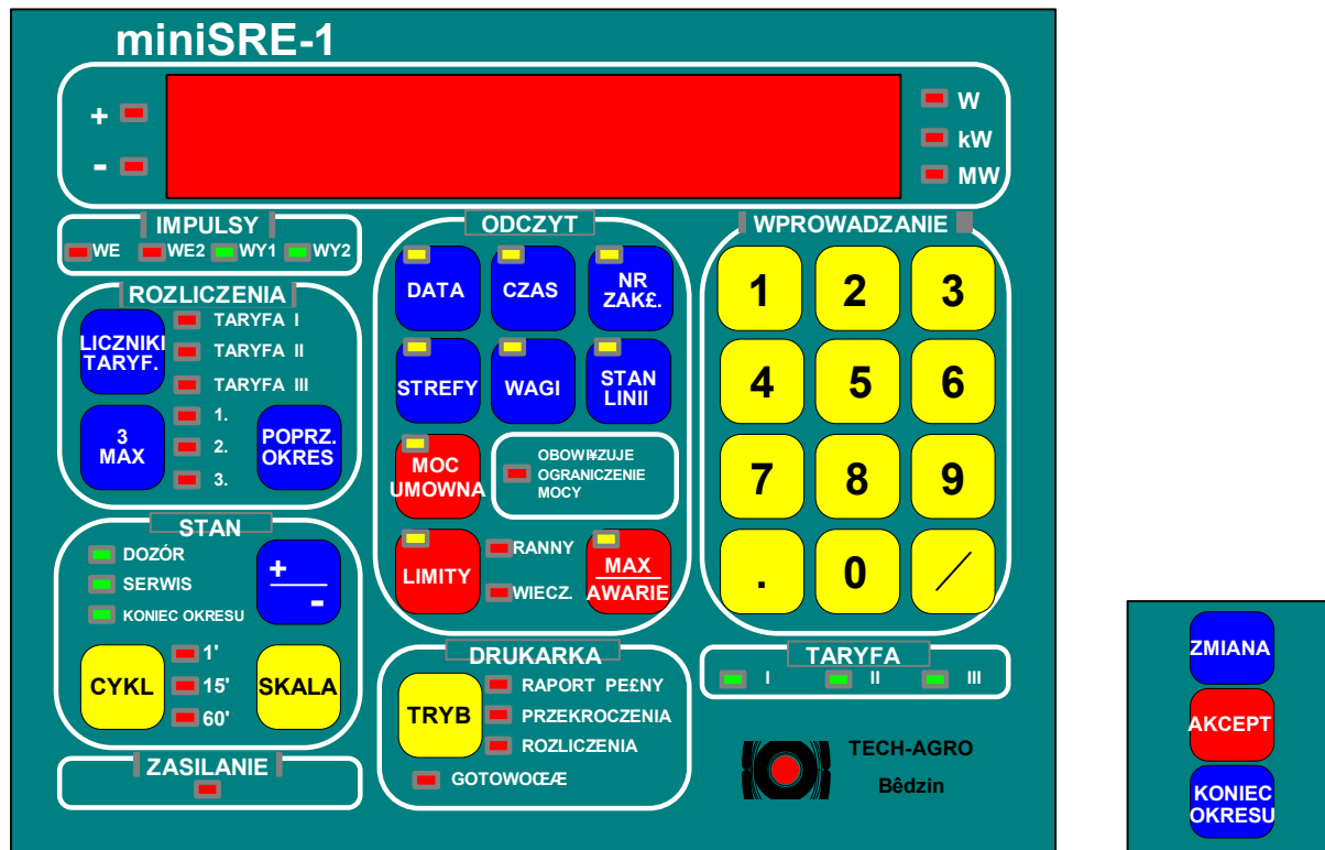
Rysunek 5. Klawiatura koncentratora miniSRE-1.
