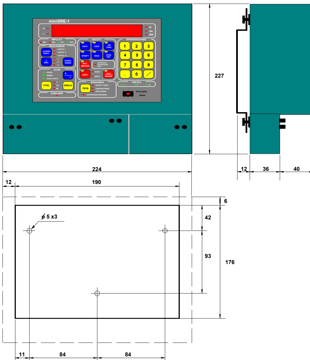
Rysunek 4. Wymiary koncentratora miniSRE-1 oraz płyty nośnej.
